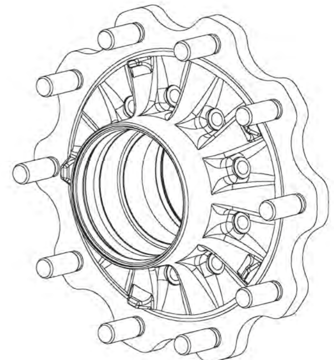
EXAMPLE OF STAR SHAPED HUB BEISPIEL EINER STERNFÖRMIGEN RADNABE
