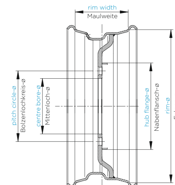
SCHEIBENRAD FÜR EINZELMONTAGE MIT 15° STEILSCHULTERFELGE FÜR SCHLAUCHLOSE BEREIFUNG
