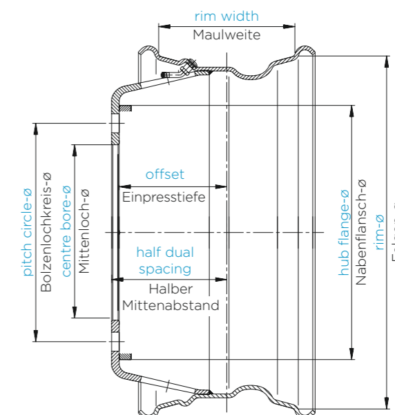
alive SCHEIBENRAD FÜR ZWILLIGSMONTAGE MIT 15° STEILSCHULTERFELGE FÜR SCHLAUCHLOSE BEREIFUNG
