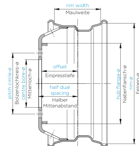
SCHEIBENRAD FÜR ZWILLIGSMONTAGE MIT 15° STEILSCHULTERFELGE FÜR SCHLAUCHLOSE BEREIFUNG
